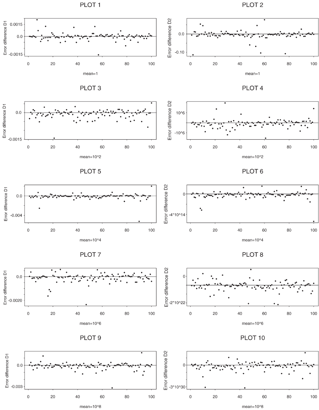
Fig. 2. n = m = 20 , B = 50 , d = 1 .
